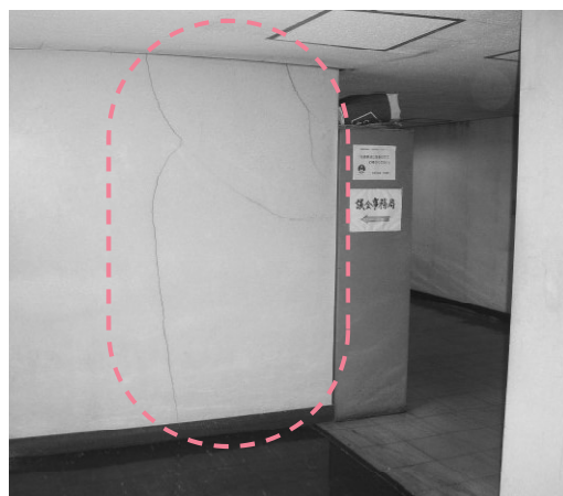
庁舎内のクラック
