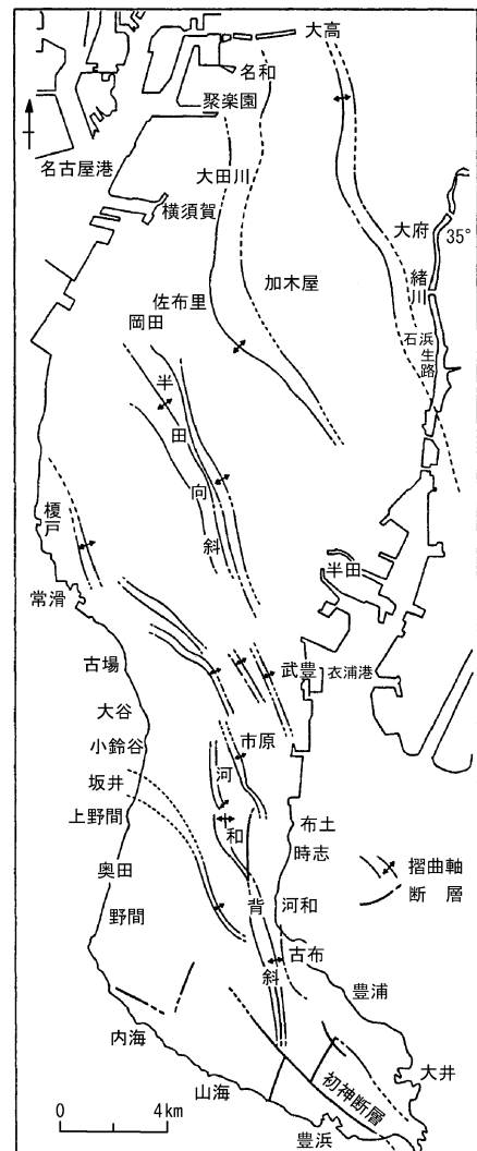
知多半島の地形構造
