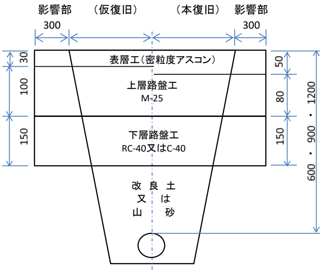
町道アスファルト舗装(L交通)
