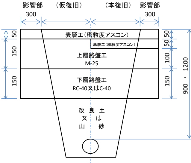
町道アスファルト舗装(B交通)
