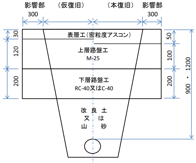
町道アスファルト舗装(A交通)
