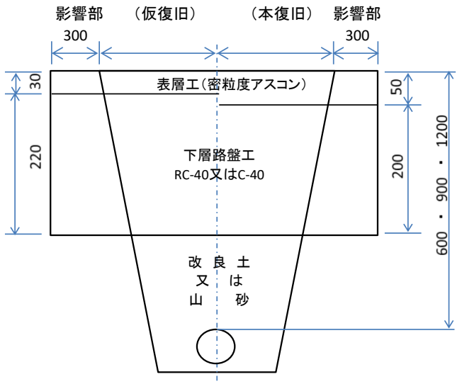
町道アスファルト舗装(簡易舗装)
