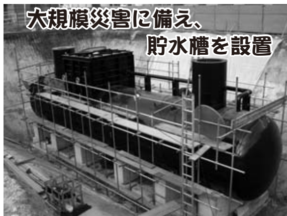
エスパランス丸山駐車場地下に設置した貯水槽
