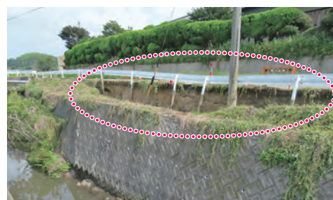
鎌子川の護岸崩壊
