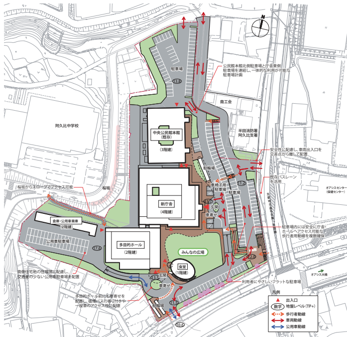
動線計画配置図
