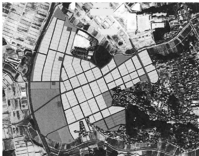
阿久比・矢高地区土地改良事業計画案（平成9年）
